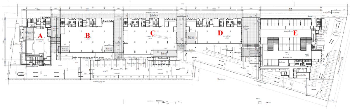
รูปภาพ 3.3.1-3 การออกแบบกลุ่มอาคารสำนักงาน ซีริ แคมปัสแนวขวาง
